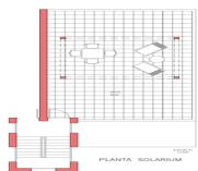
PLANTA SOLARIUM SUP. UTIL : 55,50 M2. SUP. CONSTRUIDA: 92,30 M2. SUP. DE TERRAZA DESDE: 11,00 M2. SUP. DE CUBIERTA : 60,20 M2.
